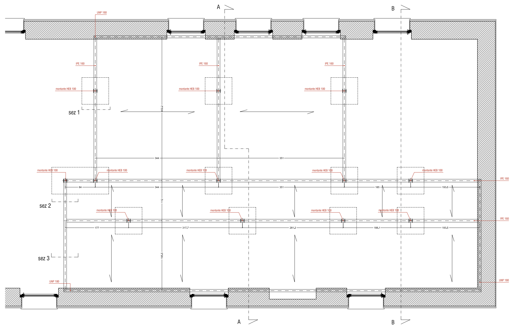
pianta carpenteria metallica
